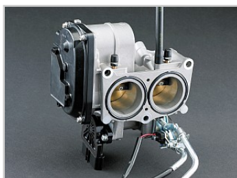
ETV-system (elektronisk trottelventil)
