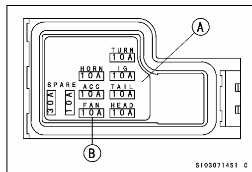
Fig.2 Säkringsdosans lock
